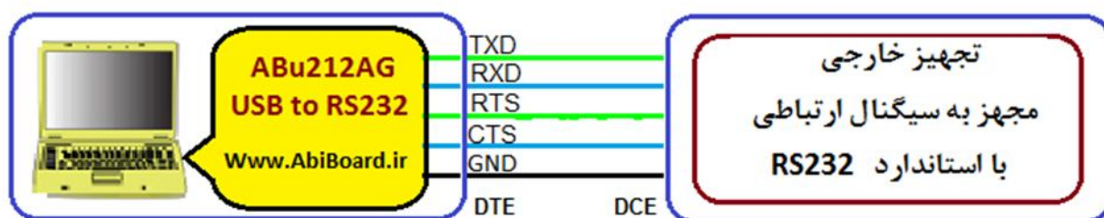
اتصال Straight مبدل به دستگاه DCE با سطح ولتاژ RS232 به همراه Handshaking
