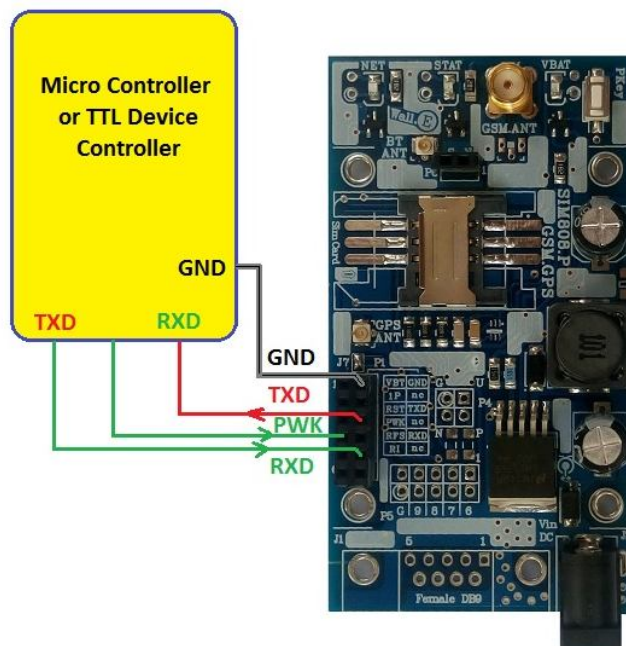
شکل 9: اتصال برد توسعه ABg184P-C به میکروکنترلر
