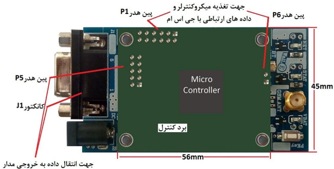
شکل 10: طراحی و نصب برد کنترل
