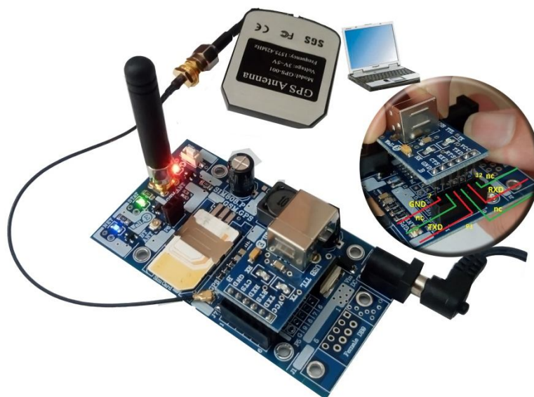
شکل 2: اتصال برد توسعه ABg184P-C به رایانه توسط مبدل یو اس بی
